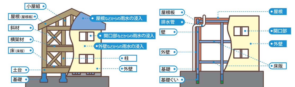
木造(在来軸組工法)の戸建住宅 (例) 2階建ての場合の骨組み(小屋組、軸組、床組)等の構成
